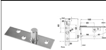
Punto de giro para herraje superior.
