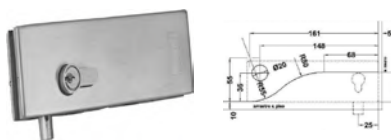
Chapa a piso con resaque. Acabado: Satín y cromo.
