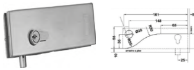
Chapa a piso con resaque. Acabado: Satín y cromo.
