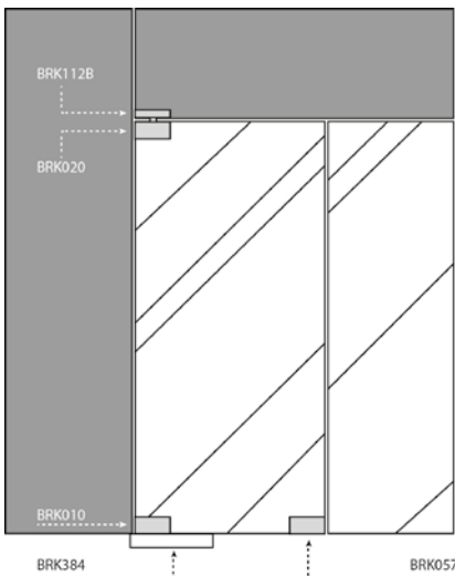
Herraje superior para punto de giro superior. Acabado: Satín y cromo.
