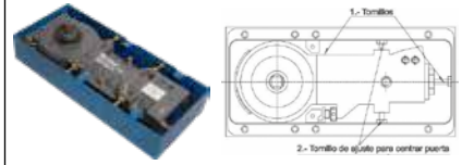
Bisagra hidráulica para 80 kg. • Material cubierta: Acero inoxidable. • Acabado: Satín. • Medidas: Perforación de piso 268mmx113mmx50mm.
