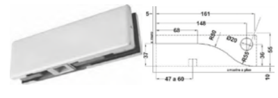
Herraje inferior para bisagra hidráulica. Acabado: Satín y cromo.
